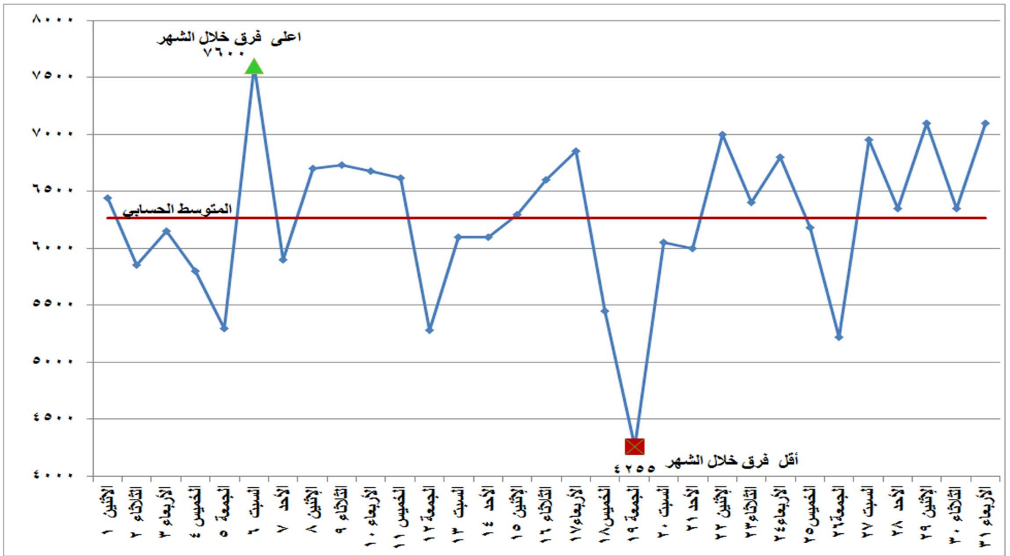
شكل (٣) الفرق بين أقصى وأدنى حمل خلال شهر يوليو ٢٠١٩
