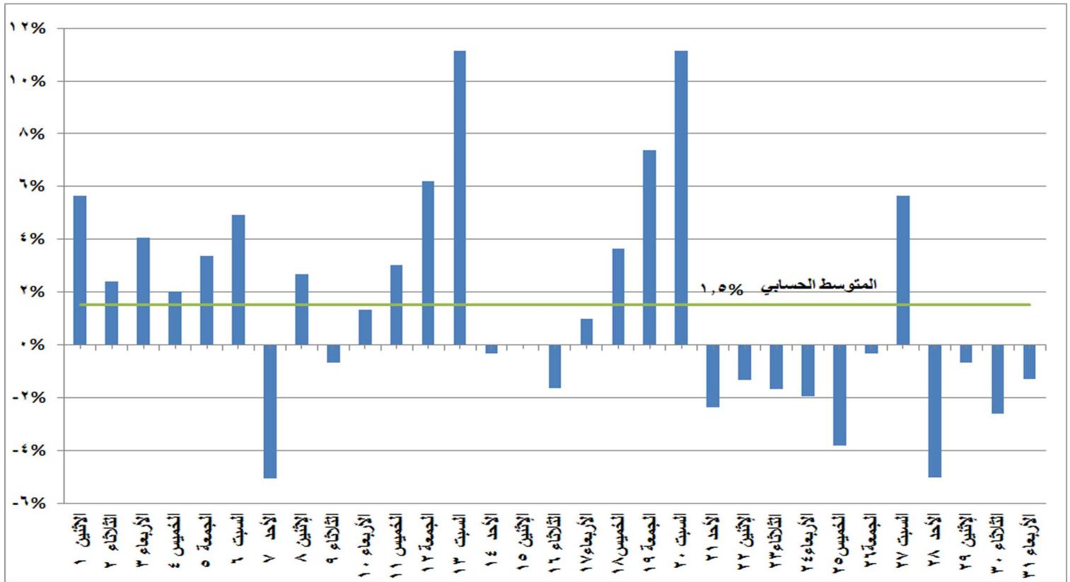
شكل (٩) النسب المئوية للتغير في الحمل الاقصى خلال شهر ٢٠١٩ مقارنة باليوم المماثل من العام الماضي
