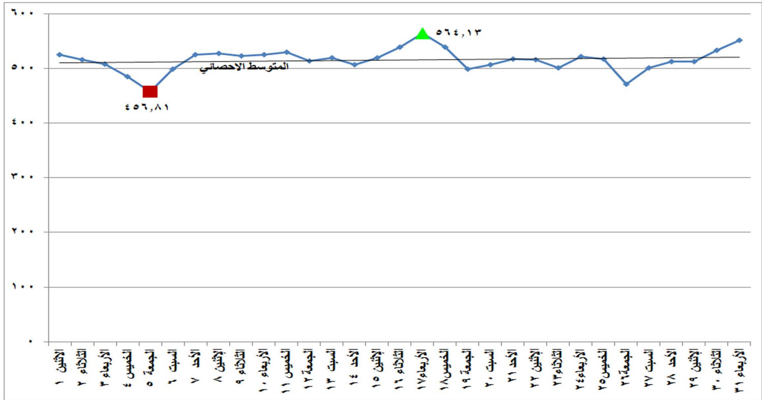
شكل (١٧) الطاقة الكهربائية المنتجة من الغاز الطبيعي خلال شهر يوليو ٢٠١٩
