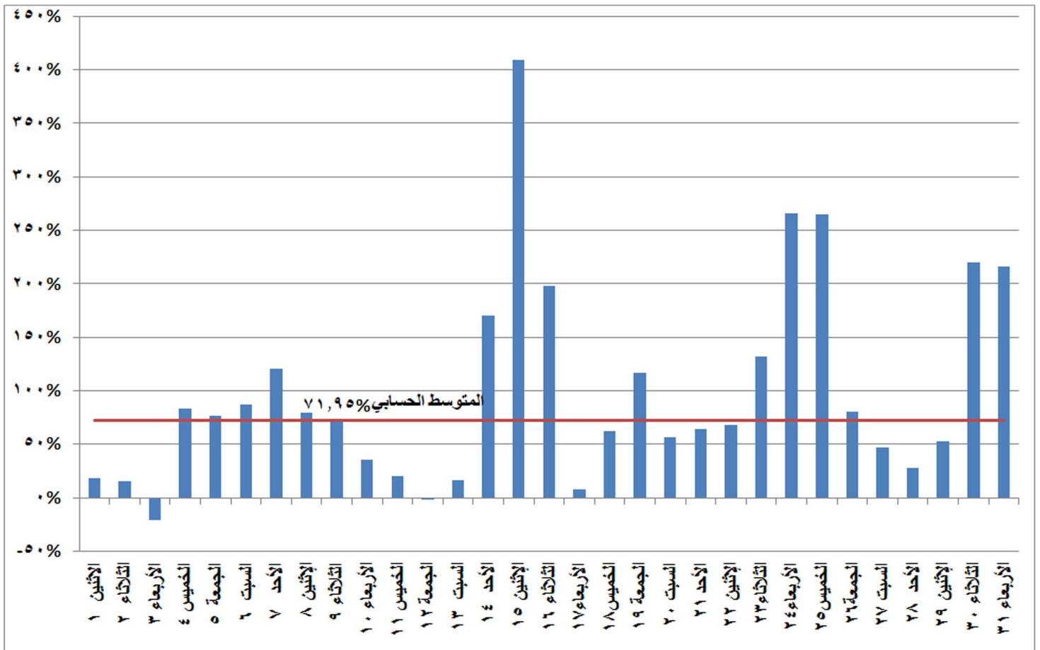
شكل (٢٦) نسب التغير في استخدام الرياح والشمس في إنتاج الطاقة الكهربائية خلال شهر يوليو ٢٠١٩ مقارنة بالشهر المماثل من العام السابق
