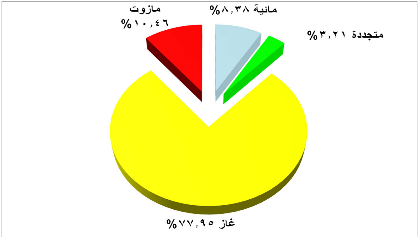
شكل (١٣) متوسط نسب مشاركة مصادر الطاقة الاولية في انتاج الكهرباء خلال شهر يوليو ٢٠١٩
