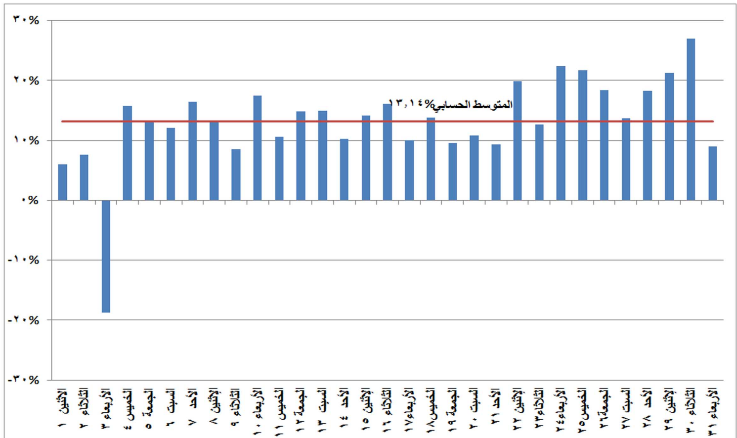
شكل (٢٤) نسب التغير في استخدام المصادر المائية في إنتاج الطاقة الكهربائية خلال شهر يوليو ٢٠١٩ مقارنة بالشهر المماثل من العام السابق
