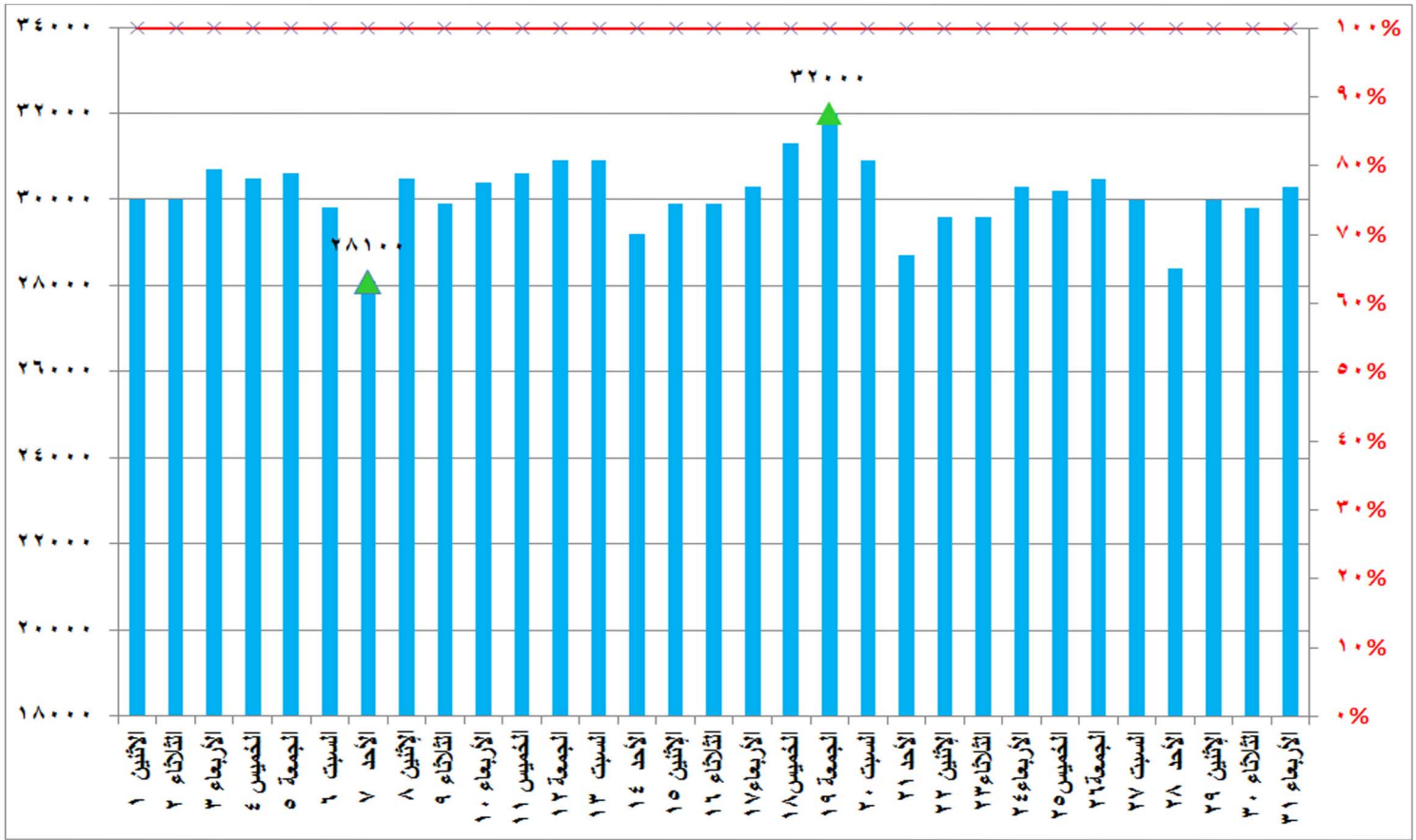
شكل (٥) قدرات الانتاج المتاحة ونسبتها للحمل الأقصى خلال شهر يوليو ٢٠١٩
