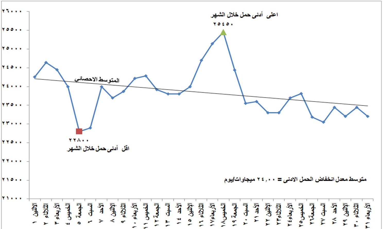
شكل (٢) تطور الحمل الادنى اليومي خلال شهر يوليو ٢٠١٩
