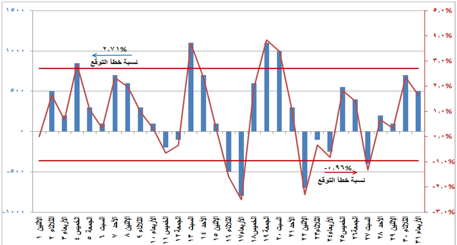
شكل (١٠) الفرق بين الحمل الأقصى المتوقع والمسجل فعليا ونسبة الفرق إلى الحمل المسجل فعليا خلال شهر يوليو ٢٠١٩
