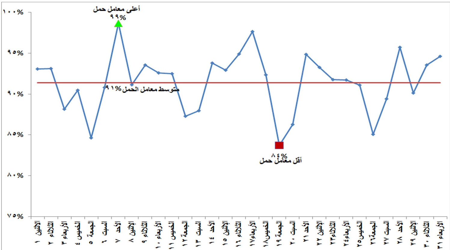
شكل (١٢) إجمالي معامل الحمل لوحدات الانتاج خلال شهر يوليو ٢٠١٩
