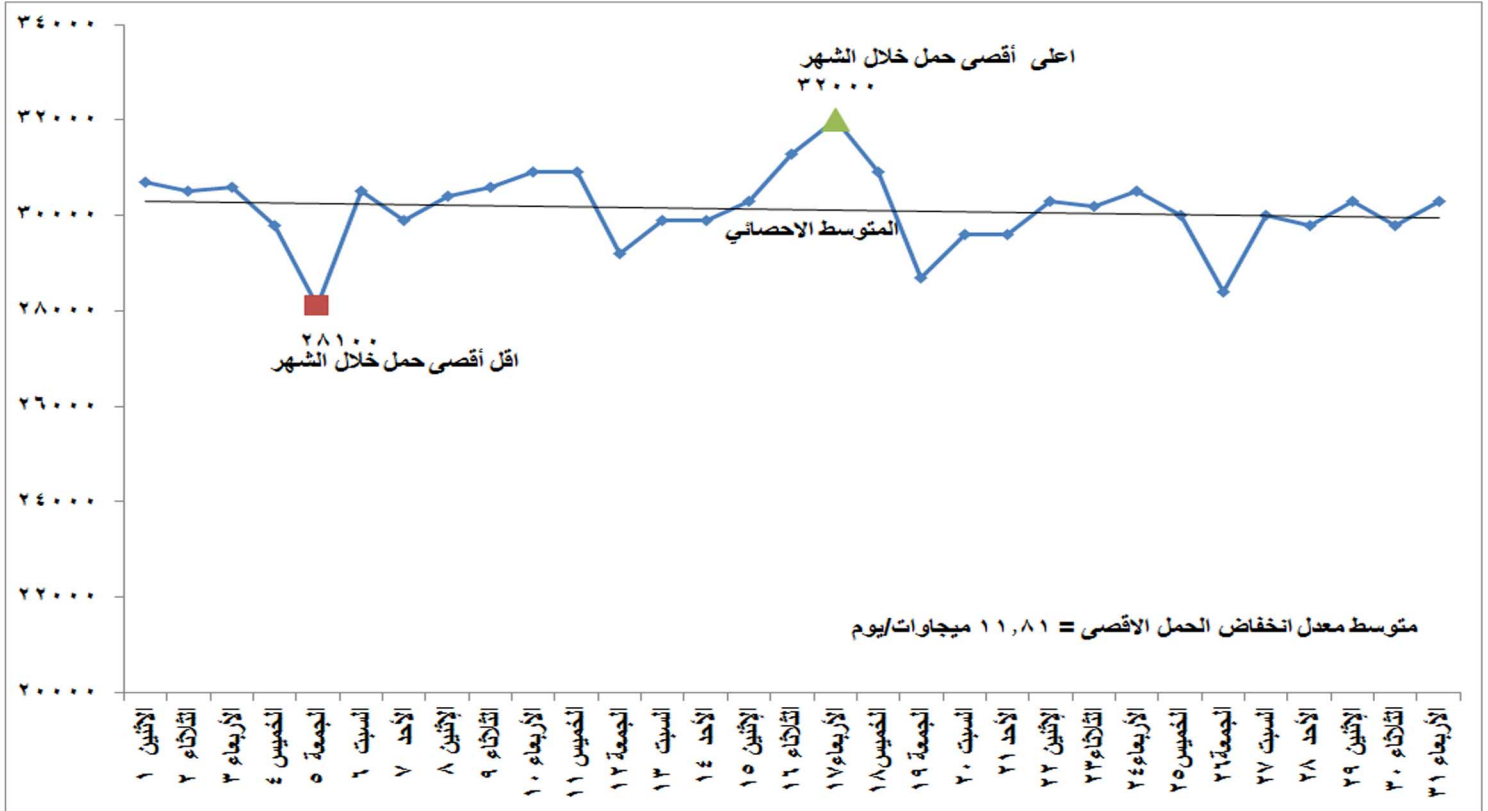
شكل (١) تطور الحمل الاقصى اليومي خلال شهر يوليو ٢٠١٩
