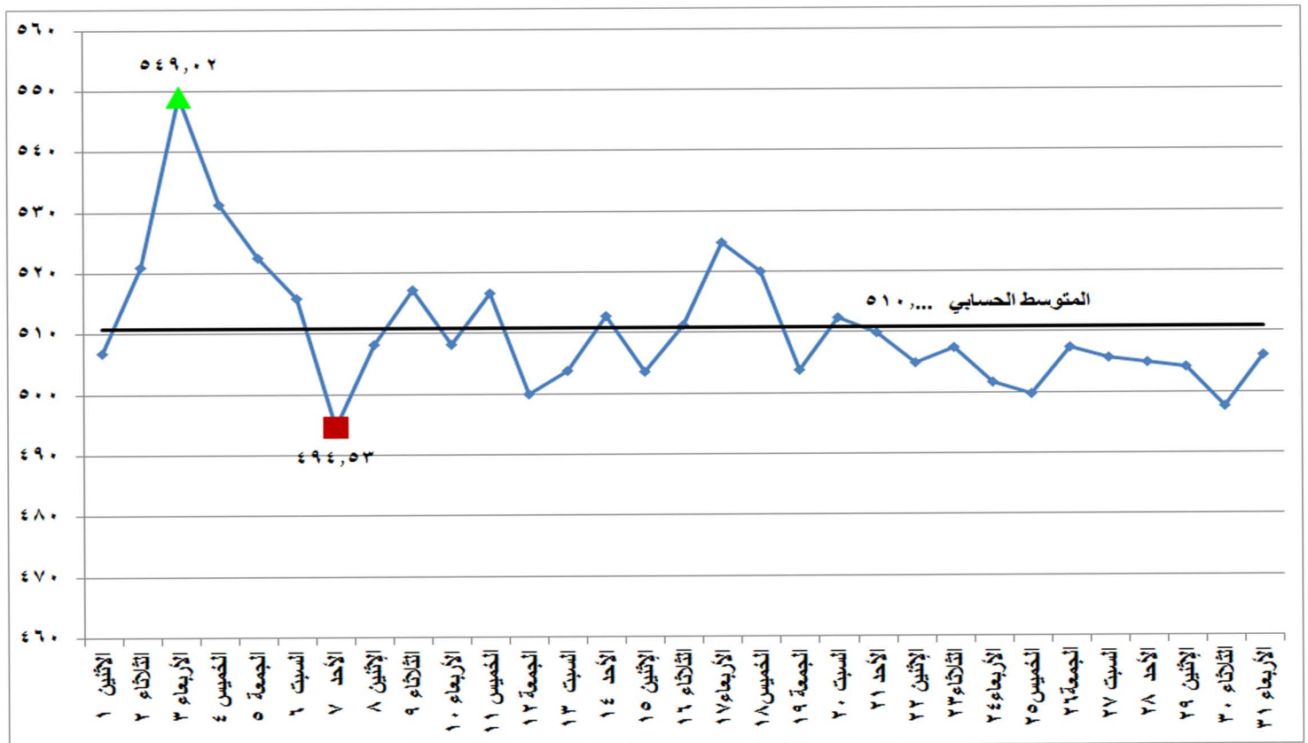
شكل (١٤) معامل انبعاثات غاز ثاني اكسيد الكربون المكافئ على مدى شهر يوليو ٢٠١٩
