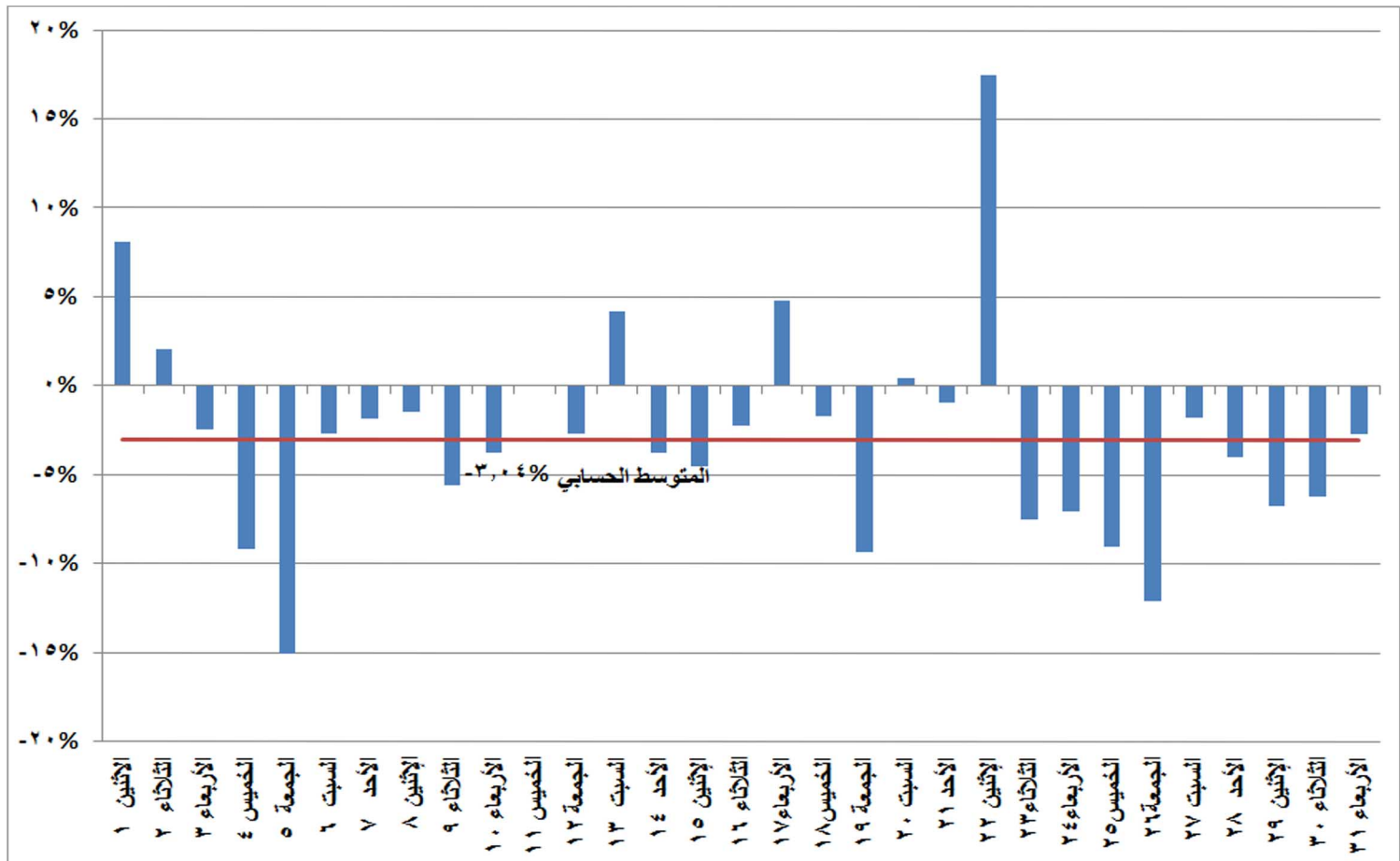
شكل (١٨) نسب التغير في استخدام الغاز الطبيعي في إنتاج الطاقة الكهربائية خلال شهر يوليو ٢٠١٩ مقارنة بالشهر المماثل من العام السابق
