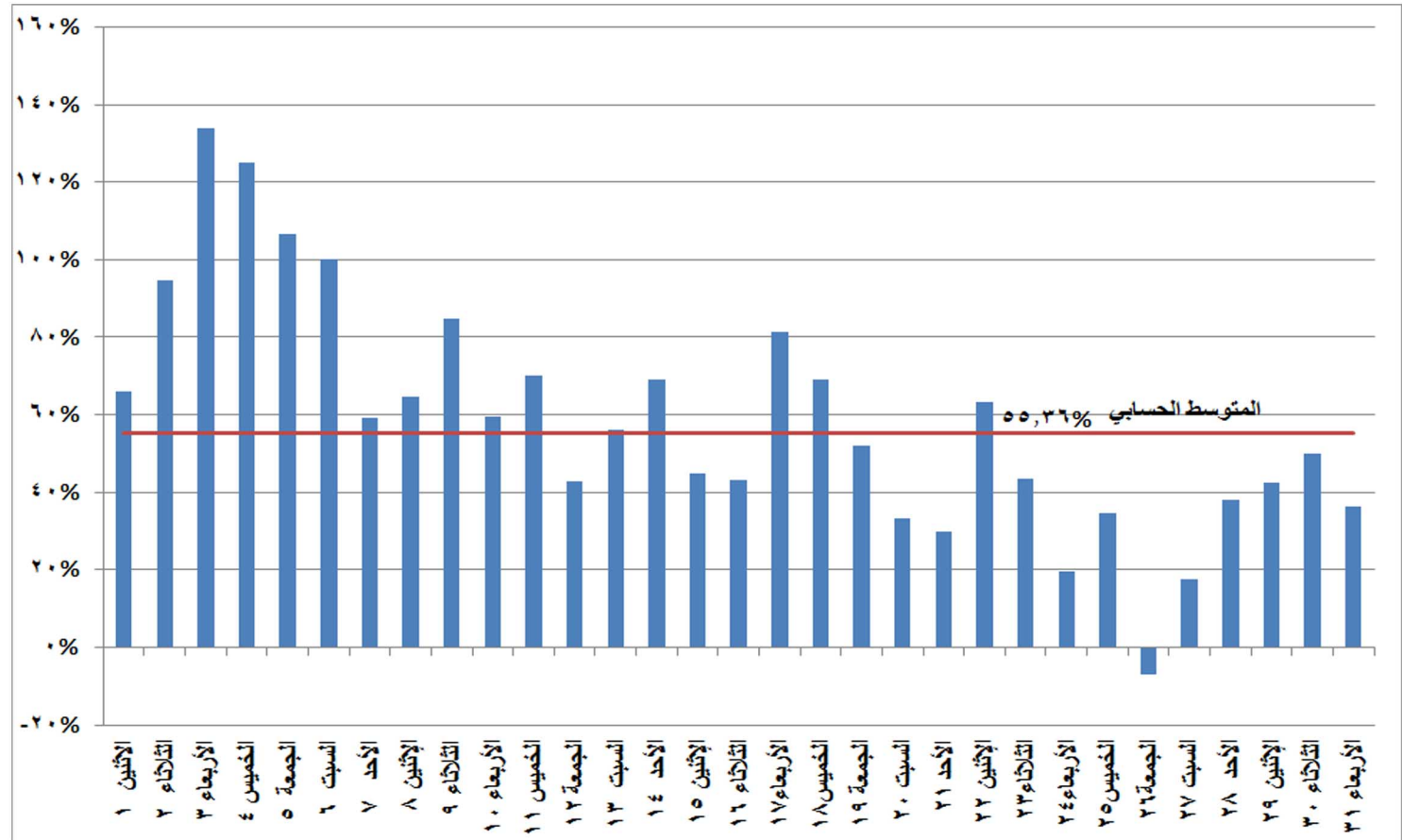
شكل (٢٠) نسب التغير في استخدام المازوت في إنتاج الطاقة الكهربائية خلال شهر يوليو ٢٠١٩ مقارنة بالشهر المماثل من العام السابق
