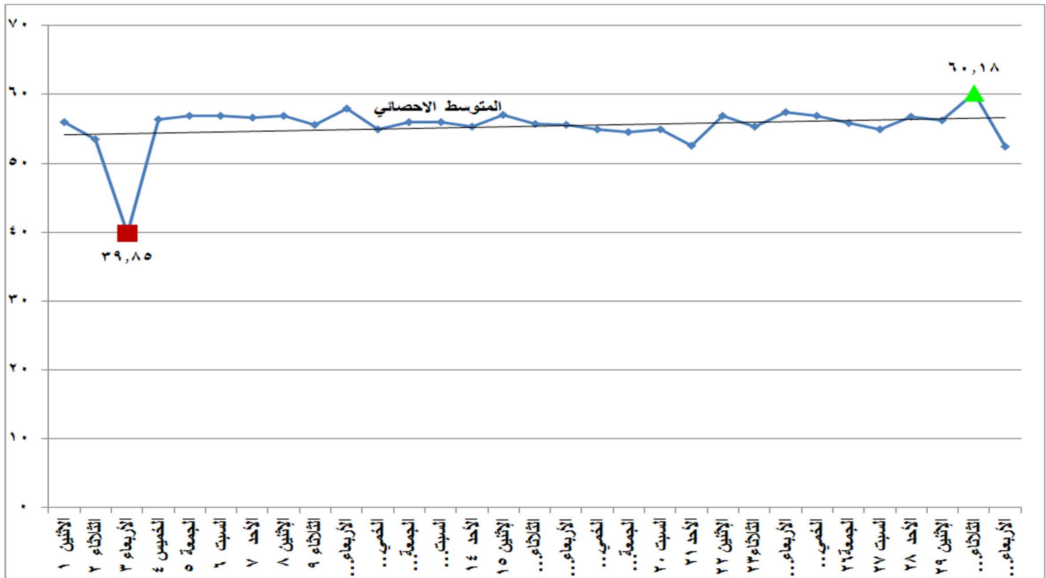
شكل (٢٣) الطاقة الكهربائية المنتجة من المصادر المائية خلال شهر يوليو ٢٠١٩
