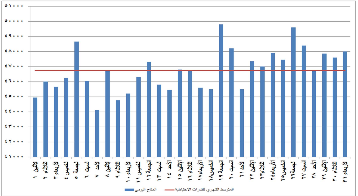
شكل (٢٧) القدرات المتاحة يوميا والمتوسط الشهري للقدرة الاحتياطية خلال شهر يوليو ٢٠١٩
